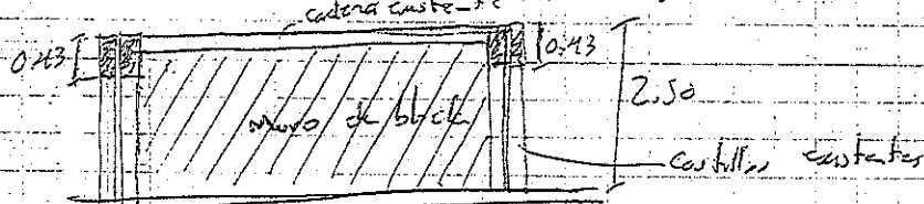
SECCION DE MURO EXISTENTE
